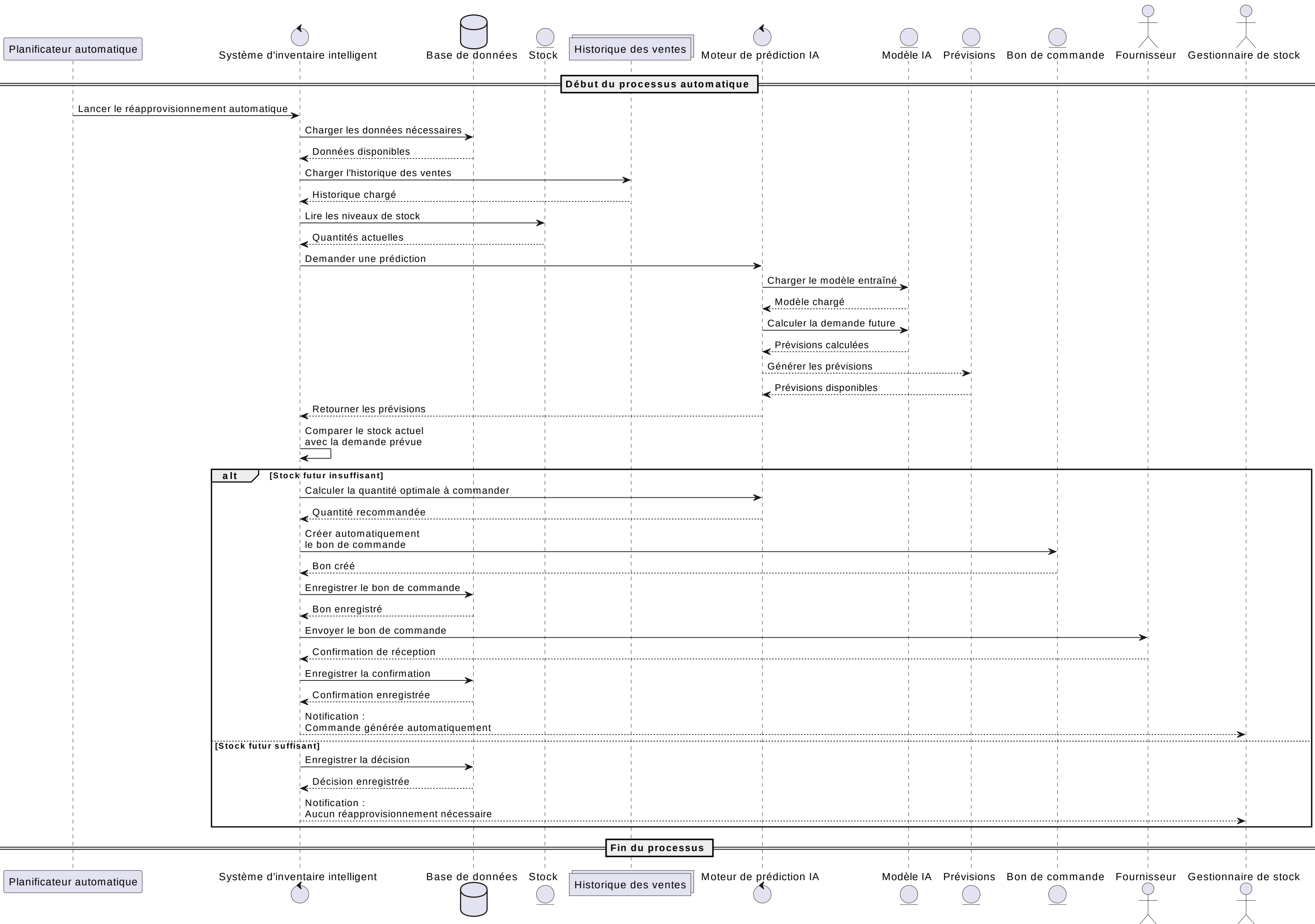
Diagramme de séquence intelligent n°5 : Réapprovisionnement basé sur la prédiction
